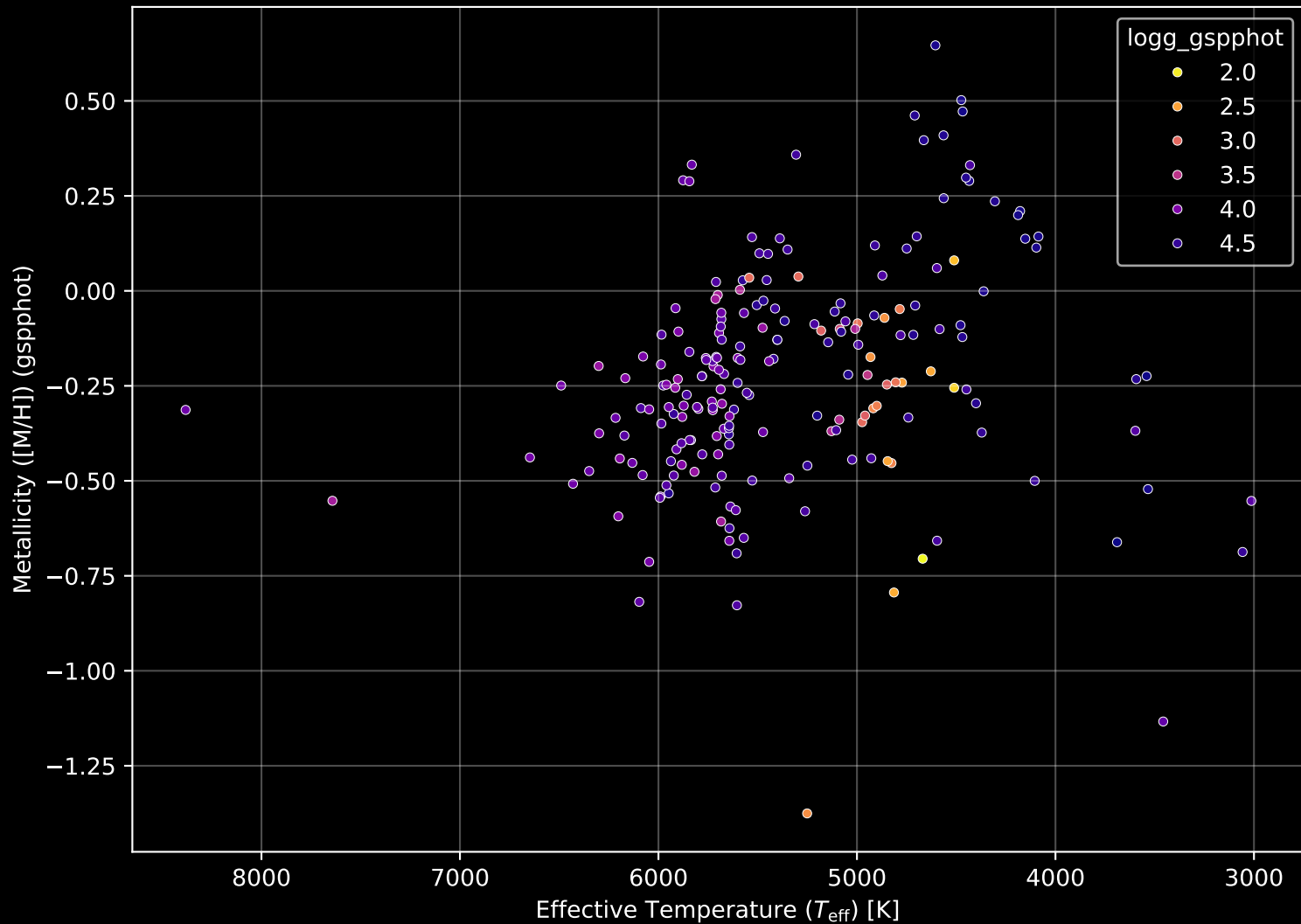
APOGEE DR17 Field: [161-57] Stellar Population Parameters (n= 207)
